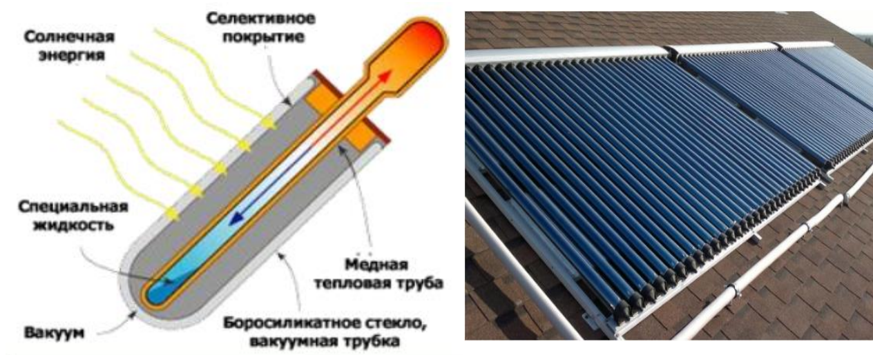
Рис. 4. Схема работы тепловой трубки.
