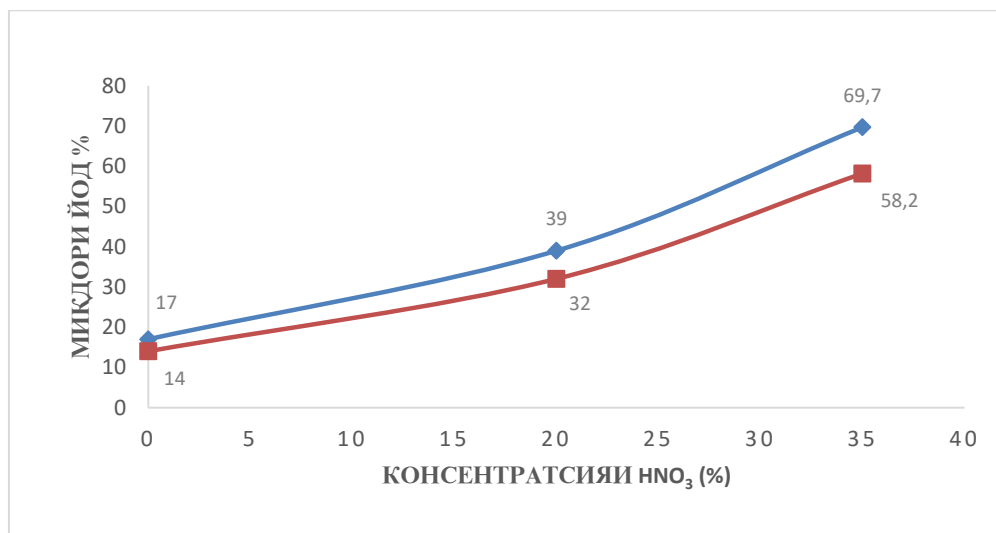
Расми 2. Вобастагии нишондоди йодии нимкокс (полукокс) аз концентратсияи кислотаи нитрат, ки барои фаълсозии сорбент истифода мешавад. Хати боло ба нимкокс (полукокс) аз ангишти «Зиддӣ», хати поён ба нимкоксии (полукокс) аз ангишти «Фон-Яғноб» ҳосилшуда мувофиқат мекунад.
