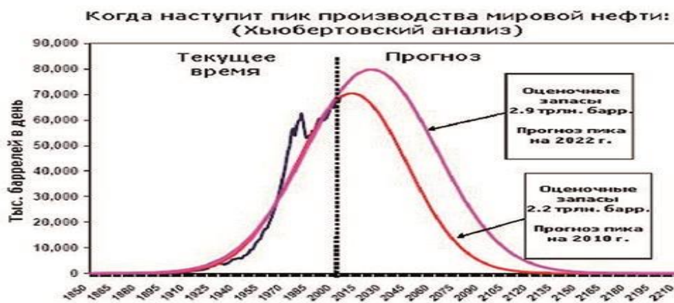
Рис. 2. Предсказание Хабберта по мировым данным
